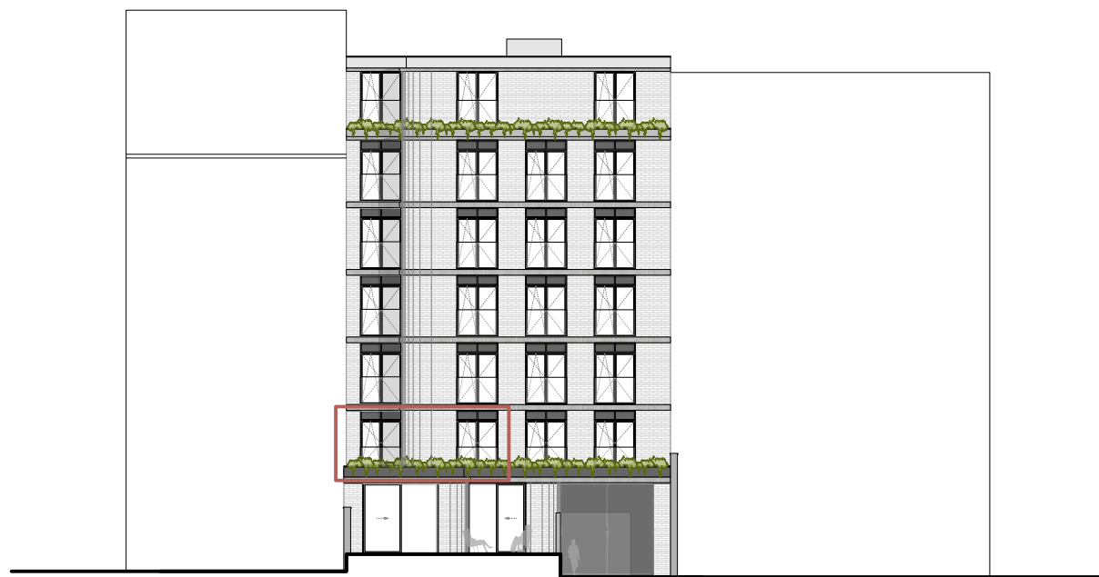
Achtergevel
